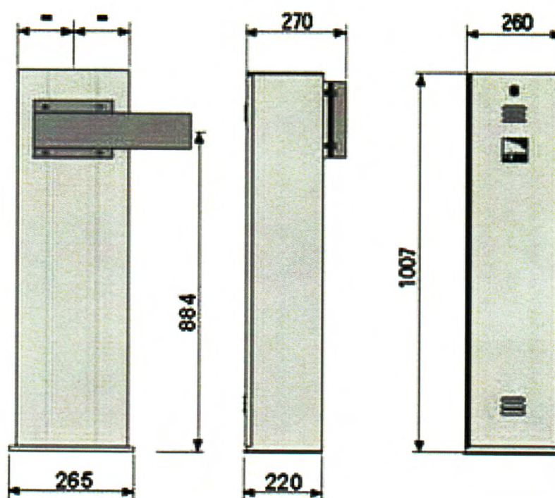
Рис. 2. Размеры шлагбаума
