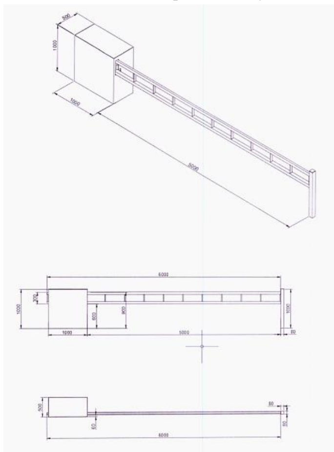
Рис. 2. Размеры шлагбаума
