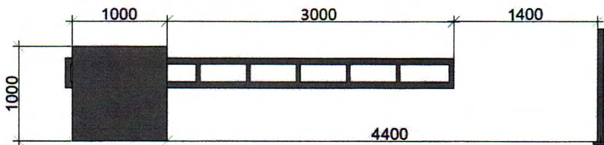
Вид сбоку
