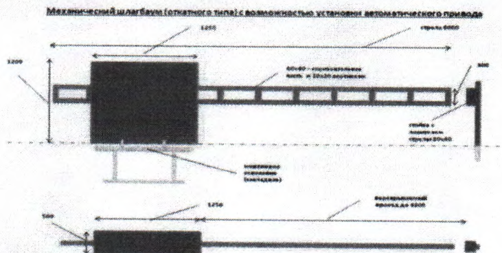
Рис. 3. Внешний вид шлагбаума
